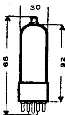
Ingombro (a)
