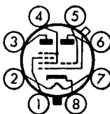
Zoccolo (b)
