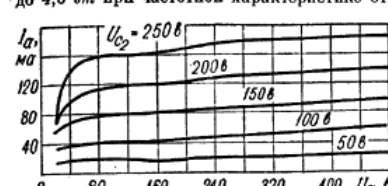
Рис. 390. Усредненные характеристики зависимости тока анода от напряжения на второй сетке 250 в: — ток в цепи анода; — — ток в цепи второй сетки; — — наибольшая мощность, рассеиваемая на аноде.
