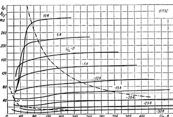
Рис. 391. Усредненные характеристики зависимости тока анода и тока второй сетки от напряжения на аноде при напряжении на второй сетке 250 в: — ток в цепи анода; — — ток в цепи второй сетки; — — наибольшая мощность, рассеиваемая на аноде.
