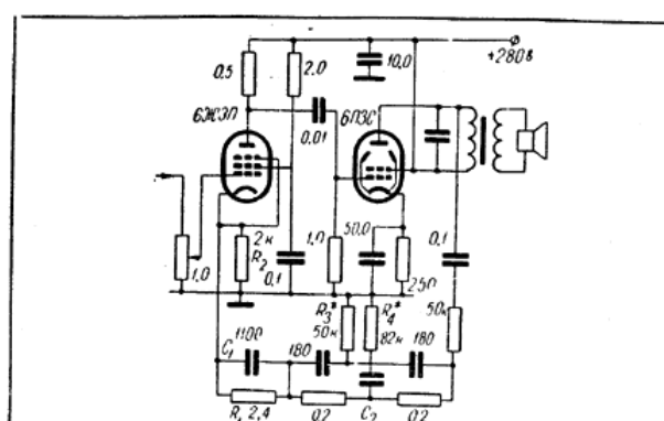
Рис. 388. Схема применения лампы 6П3С в качестве однокатного усилителя мощности низкой частоты в классе А.
