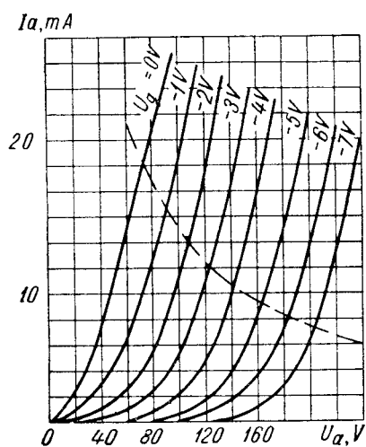
I_a = f(U_a) (каждого триода) (for each triode) — — — P_{a \max} U_h = 6,3 \text{ V}
