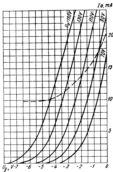
I_a = f(U_{gT}) (каждого триода) (for each triode) — — — P_{a \max} U_h = 6,3 \text{ V}
