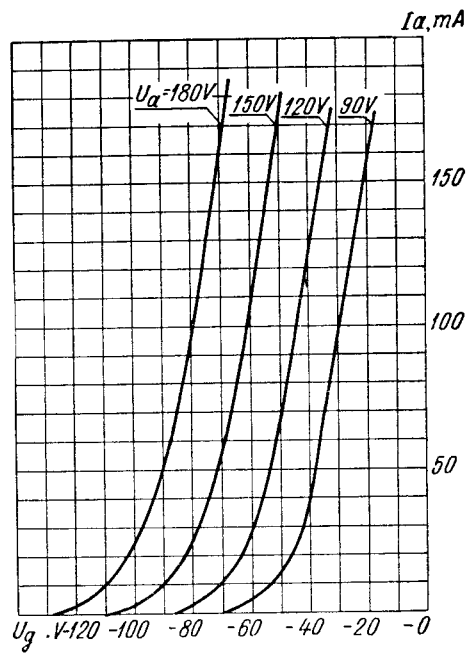
I_a = f(U_{гТ}) (каждого триода) (for each triode) U_h = 6,3 \text{ V}
