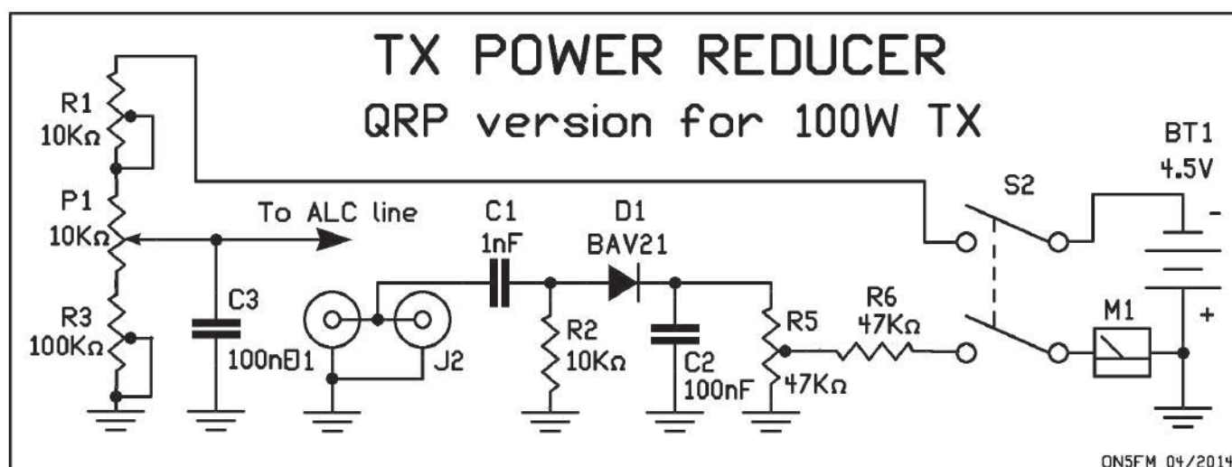
Version pour rendre QRP un TX 100 W sur simple bascule-
