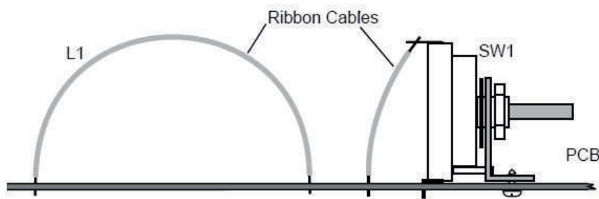
Dessin de la self et du commutateur
