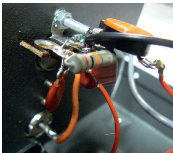
Vue du circuit wattmètre côté amphenol. On distingue R2 de 10\text{K} - 1\text{W} , la diode BAV21 et la résistance ajustable R5.
