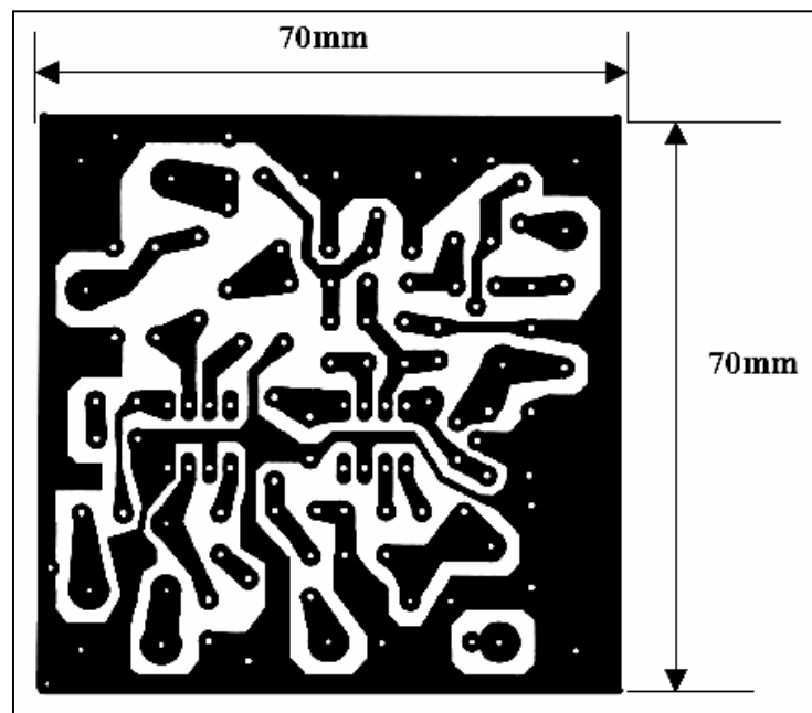
A gauche, circuit miroir côté composants. Ci-dessus, côté cuivre
