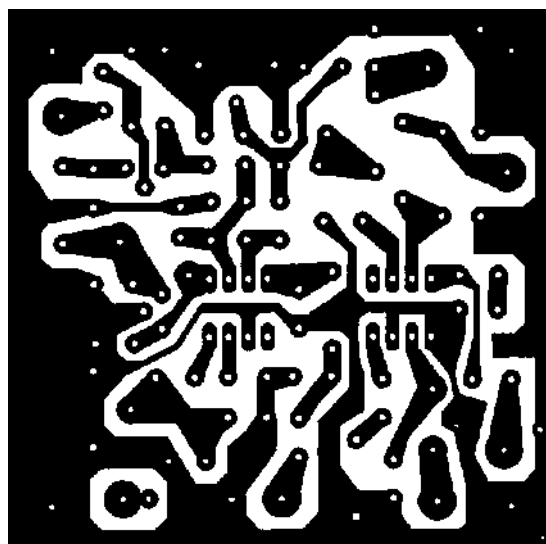
A gauche, circuit miroir côté composants. Ci-dessus, côté cuivre
