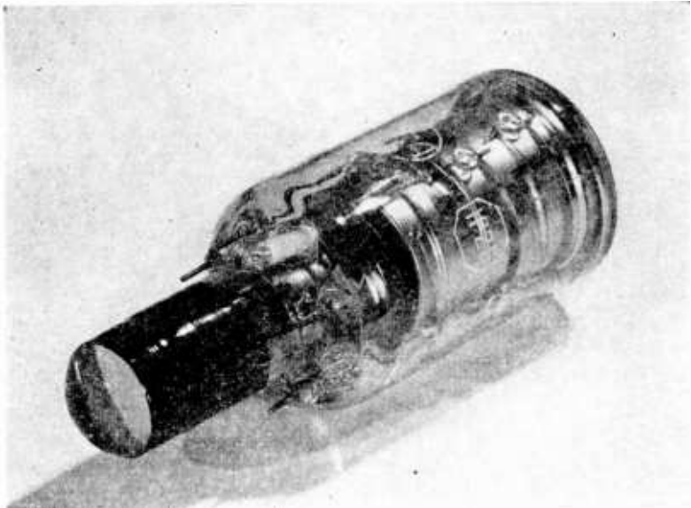
Fig. 7—1P25 Image Tube.
