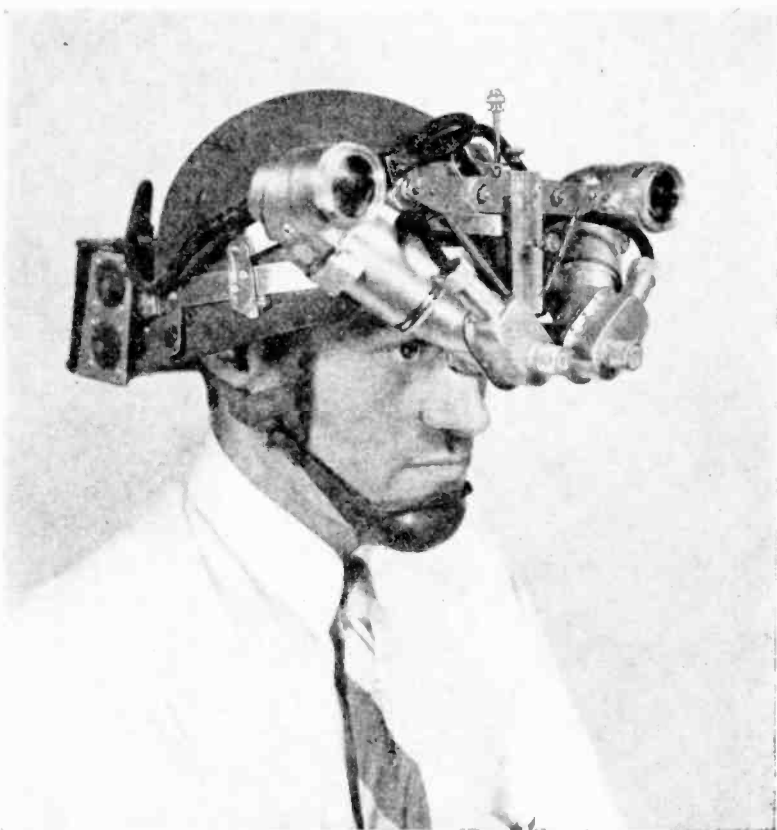
Fig. 12—Type Z Helmet Binocular.
