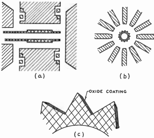
Fig. 4— Grooved cathode.
