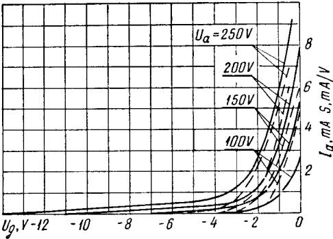
I_a, S = f(U_g) — I_a U_h = 6,3 V - - - S
