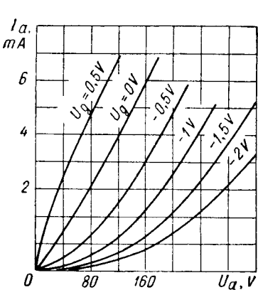
I_a = f(U_a) U_h = 6,3 V
