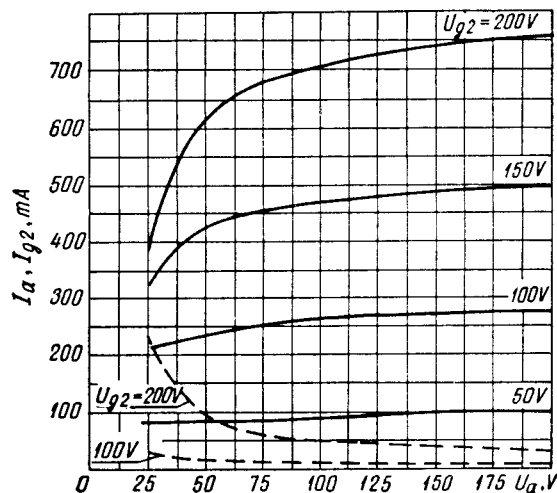
I_a, I_{g2} = f(U_a) — I_a U_h = 6,3 V - - - I_{g2} U_{g1} = 0
