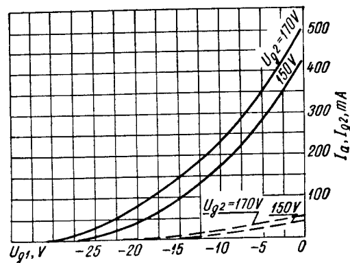
I_a, I_{g2} = f(U_{g1}) — I_a U_h = 6,3 V - - - I_{g2} U_a = 50 V
