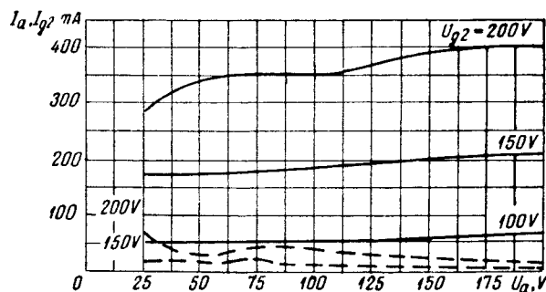
I_a, I_{g2} = f(U_a) — I_a U_h = 6,3 V - - - I_{g2} U_{g1} = -10 V
