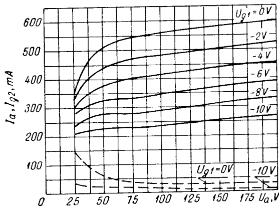
I_a, I_{g2} = f(U_a) — I_a U_h = 6,3 V - - - I_{g2} U_{g2} = 170 V
