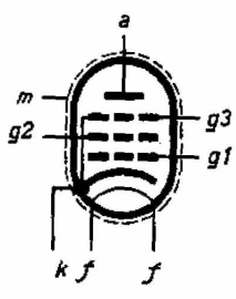
Disposition des électrodes et connexions du culot.
