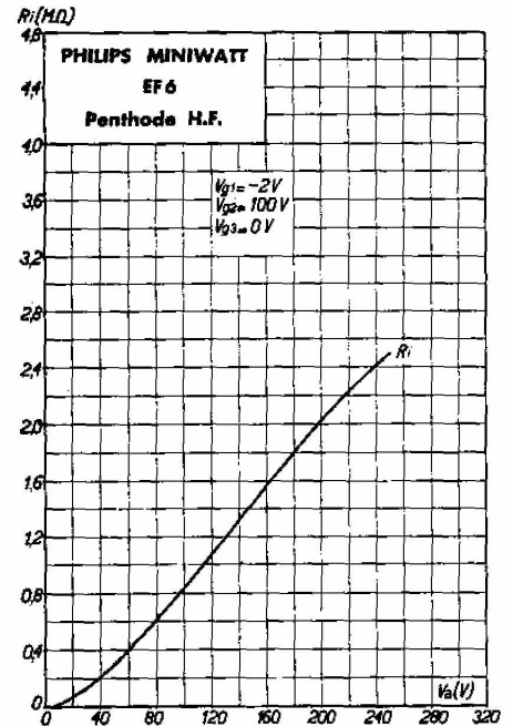
Résistance interne en fonction de la tension d'anode pour V_{g2} = 100 V et V_{g1} = -2 V.
