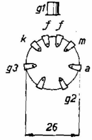
Disposition des électrodes et connexions du culot.
