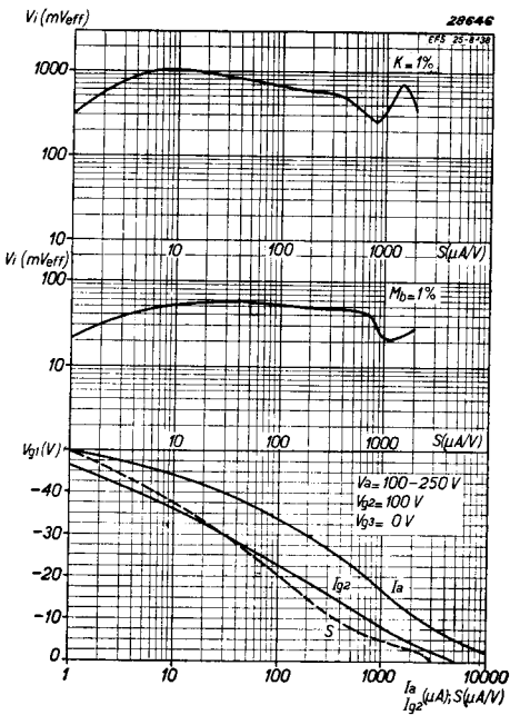
Abb. 5 Für eine Schirmgitterspannung von 100 V : Obere Kurve: Effektive Gitterwechselspannung als Funktion der Steilheit für 1 % Quermodulation. Mittlere Kurve: Effektive Gitterwechselspannung als Funktion der Steilheit für 1 % Modulationsbrummen. Untere Kurven: Steilheit S und I_a als Funktion der Spannung des ersten Gitters.
