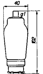
Dimensions du tube KF3.
