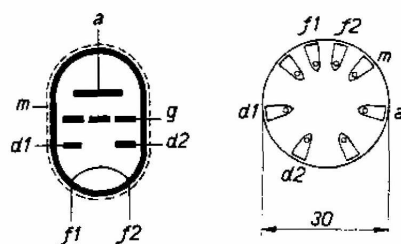
Disposition des électrodes et connexions du culor du tube KBC 1
