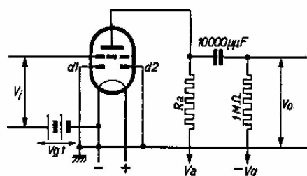
Montage du tube KBC 1 qui a servi à faire les mesures dont les résultats figurent dans le tableau.
