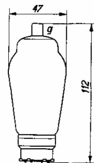
Encombrement du tube KBC 1.
