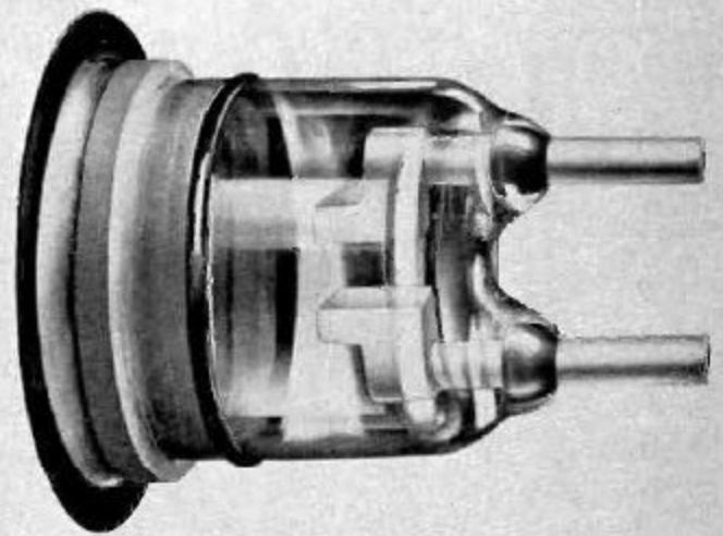
ANODE ASSEMBLY
