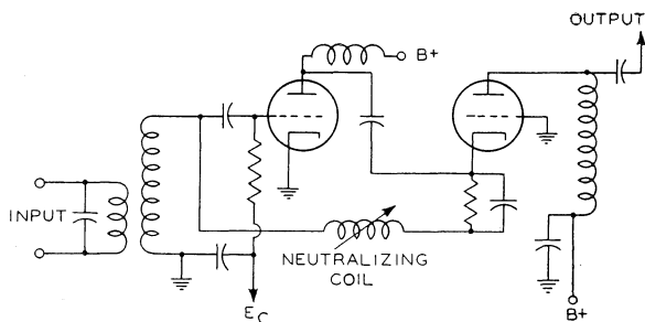
Fig. 2—Cascode circuit.
