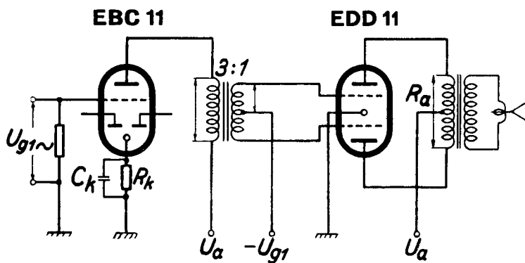
Prinzipschaltbild
