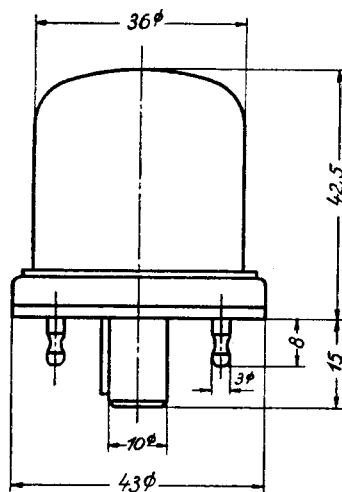
Kolbenabmessungen
