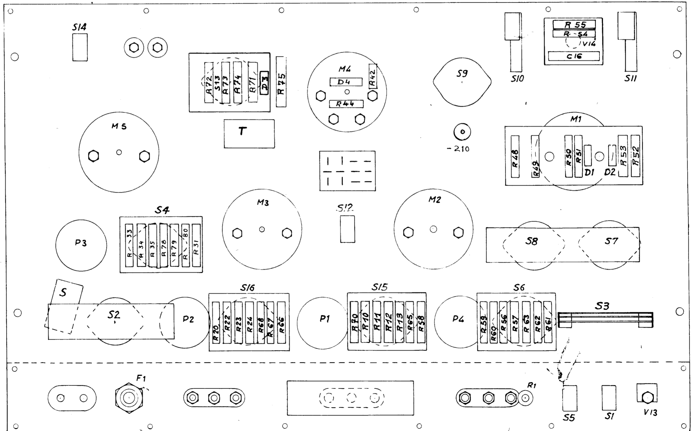
Platine principale - Vue arrière
