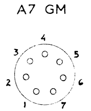
AMERICAIN 7 BROCHES GM
