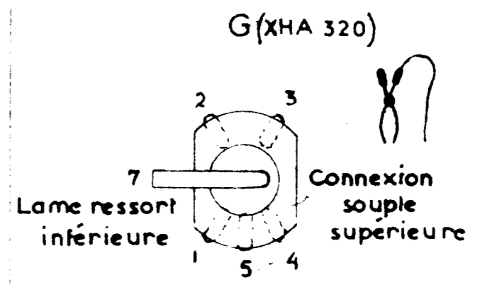
GLAND
