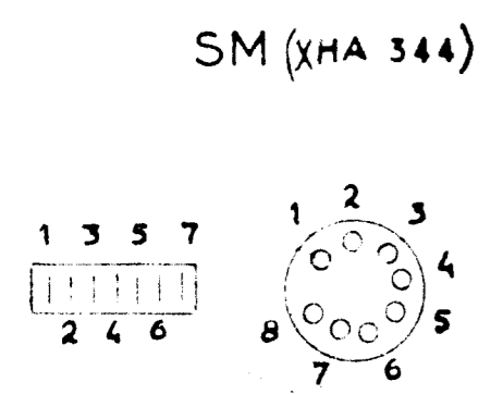
SUBMINIATURE
