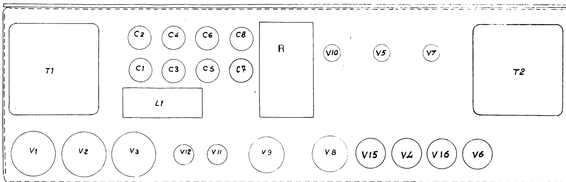
Châssis. Vue de dessus
