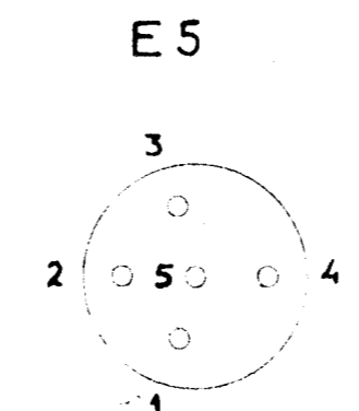
EUROPEEN 5 BROCHES
