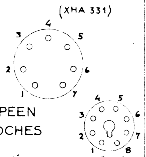
SUBMINIATURE
