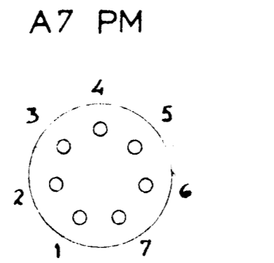
AMERICAIN 7 BROCHES PM
