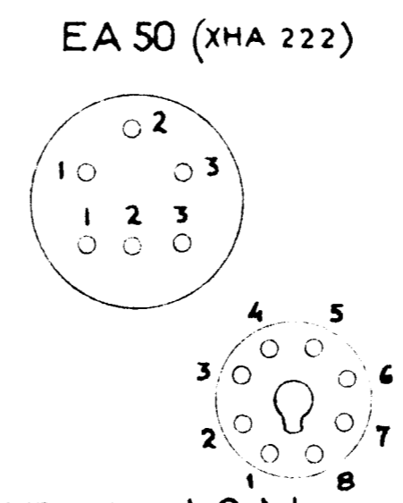
monté sur support Octal
