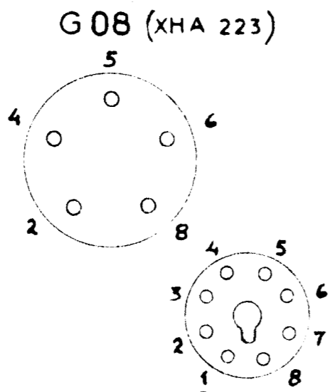
Support subminiature à vis monté sur support Octal
