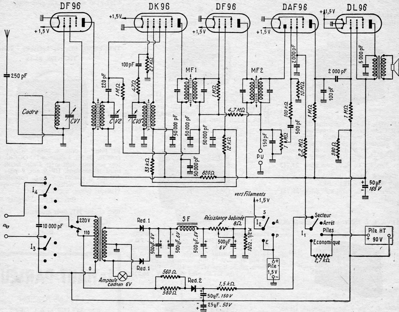
FIG. 1. — Schéma de principe complet du BIARRITZ
