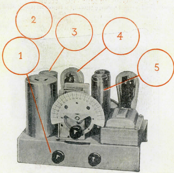
1. Circuit préselecteur ; 2. Dynamique licencié ; 3. Détectrice penthode 4. Penthode B.F. de puissance 7 W. ; 5. Double filtrage secteur. Bloc condensateur variable à air Wireless . Prise pick-up.
