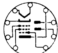
UBF89
