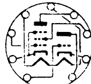
UCL82
