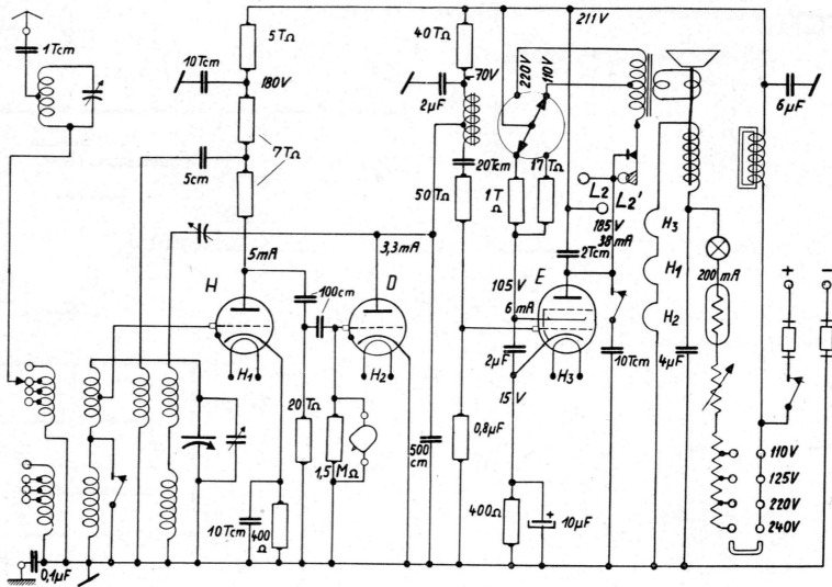
Abb. 202. Ideal, Blaupunkt 3 G 15, Gleichstrom, 1 Kreis, Gruppe 22
