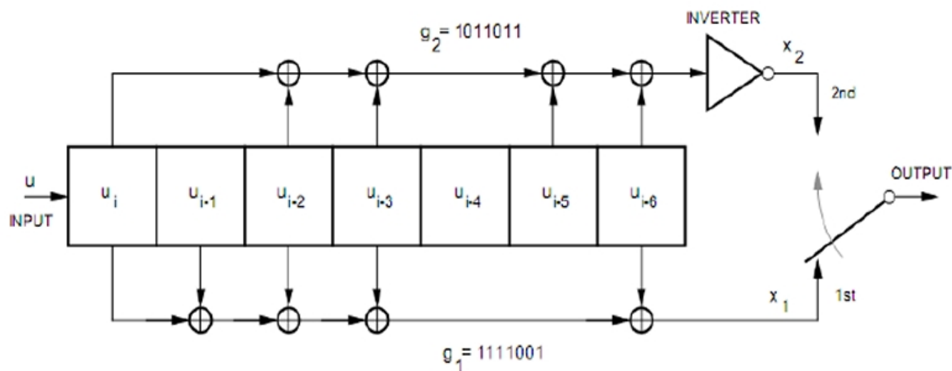
Codeur convolutionnel
