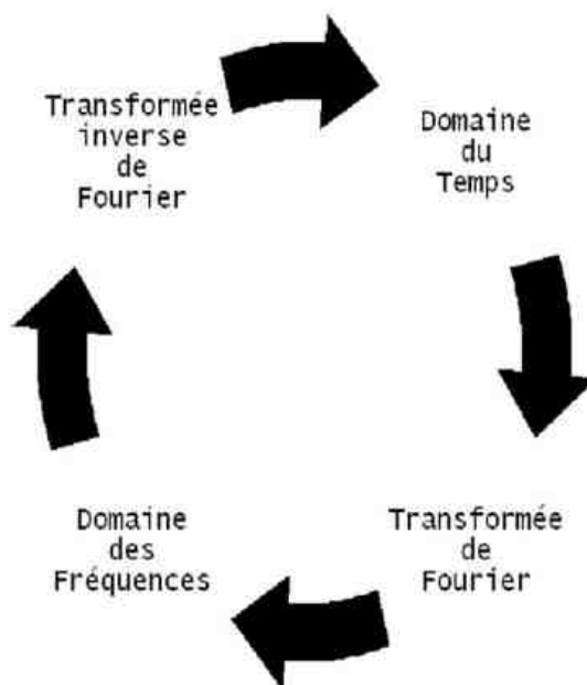
Relation entre le domaine du temps et celui des Fréquences
