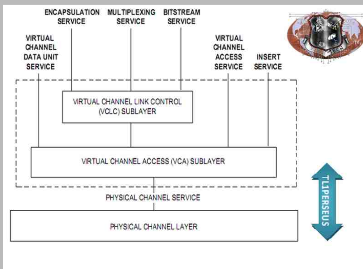
Place du système dans le modèle OSI
