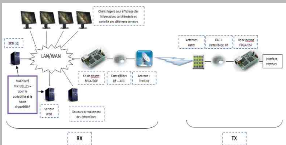
Représentation schématique de l'architecture du système final
