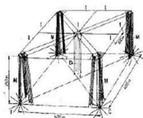
Fig. 2. - Le réseau des antennes.
