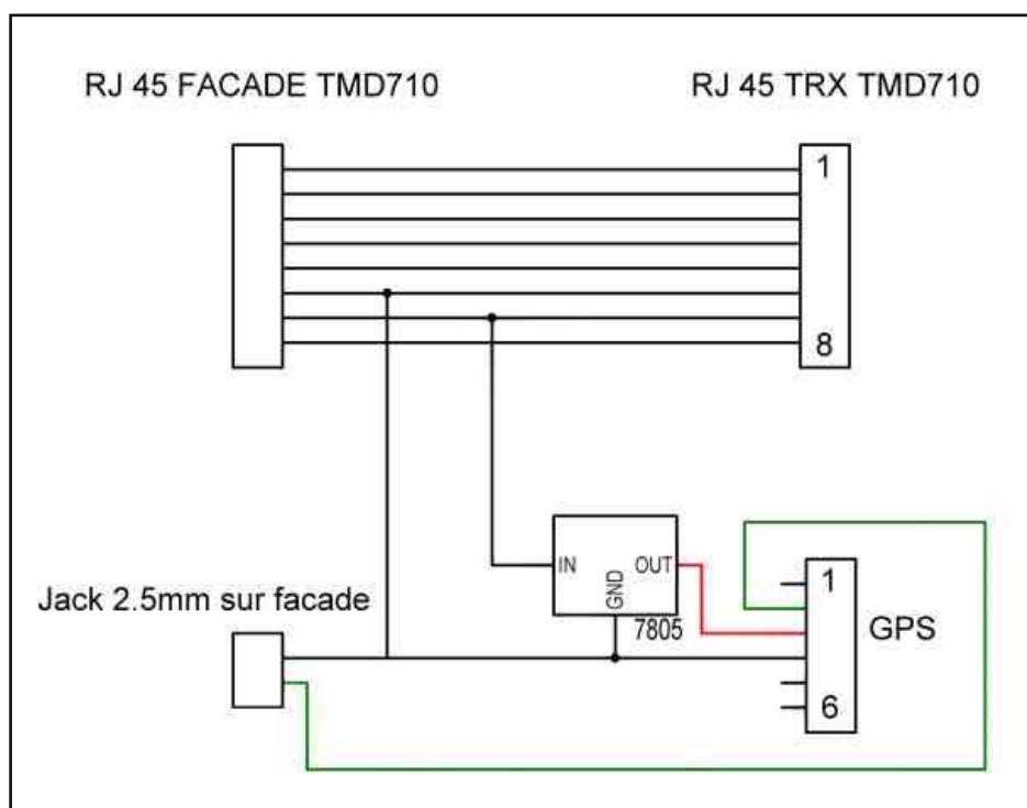
Schéma de câblage
