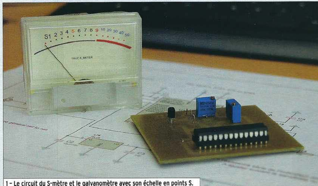
1 - Le circuit du S-mètre et le galvanomètre avec son échelle en points S.
