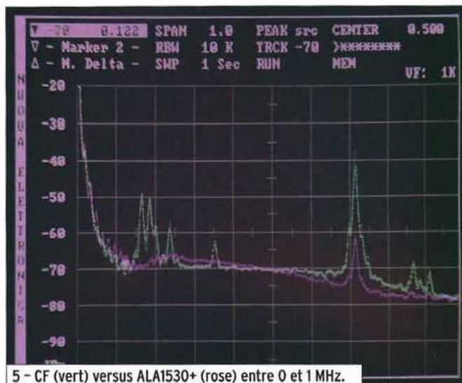
5 - CF (vert) versus ALA1530+ (rose) entre 0 et 1 MHz.
