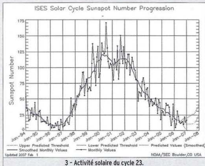
3 - Activité solaire du cycle 23.
