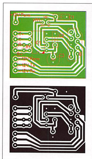
Figure 14A - Implantation composants convertisseur RS422. Figure 14B - CI convertisseur RS422.
