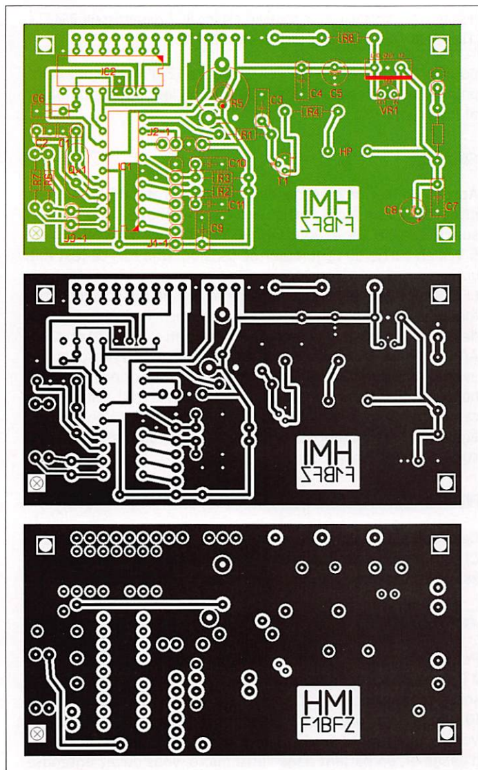
Figure 10A - Implantation composants IHM (Version B). Figure 10B - CI IHM (Version B) côté soudures. Figure 10C - CI IHM (Version B) côté composants.
