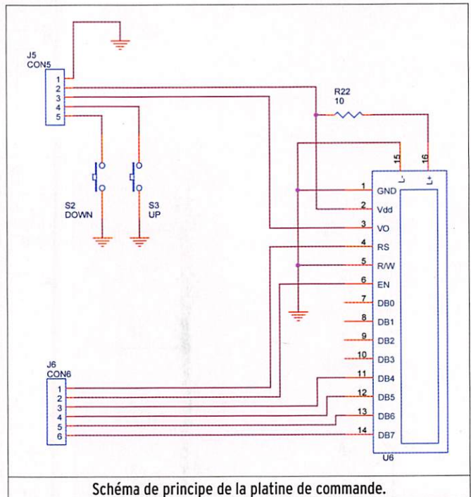
Schéma de principe de la platine de commande.
