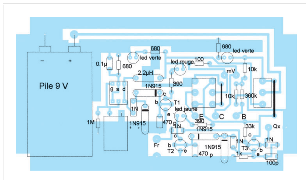
Figure 5: L'implantation des composants. Le circuit imprimé est vu en transparence.
