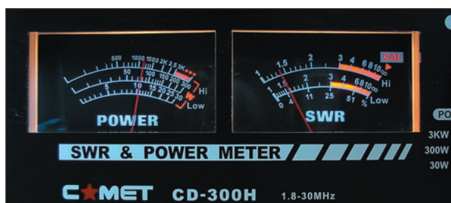
3 - Deux beaux galvas pour une lecture aisée ; ici, 75 W et 1,4/1 de ROS.
