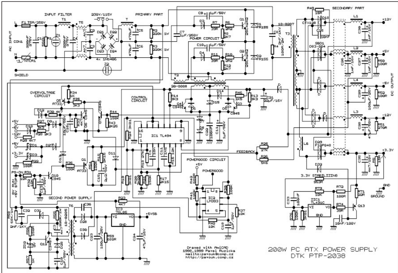
Figure 1: Schéma type d'une alimentation ATX pour PC de 200 W [4].
