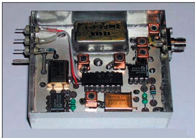
1 - Module réception PSK du satellite Echo.
