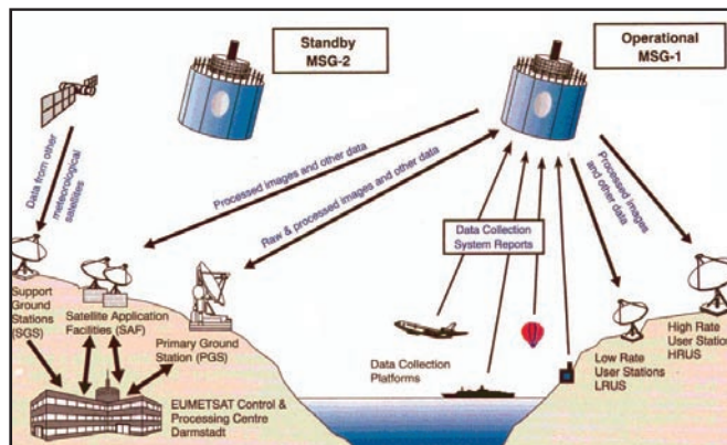
Réseau communication autour de MSG1.
