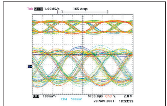
Fig.6 : Courant PLL = 200 µA, chemin de modulation d'origine, TXD = 150 ms, BER OK, œil OK.
