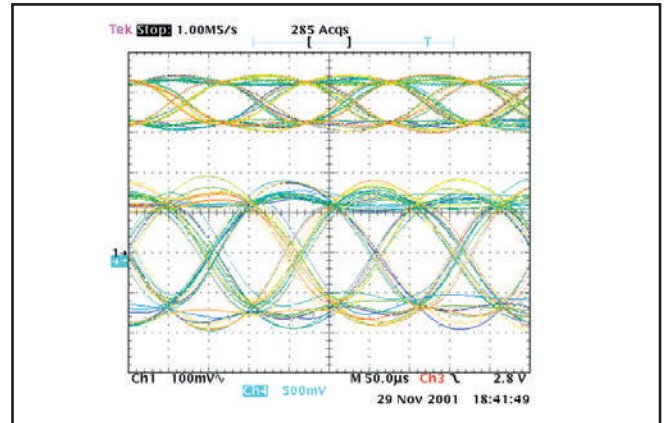
Fig.5 : Courant PLL = 100 µA, chemin de modulation d'origine, TXD = 350 ms, BER super, œil super.
