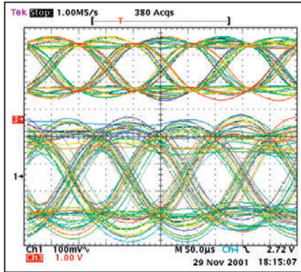
Fig.3. Diagramme de l'œil d'origine, courant du PLL = 800 µA, TXD = 150 ms. En haut l'œil du TX, en bas celui du RX -- pas très bons.
