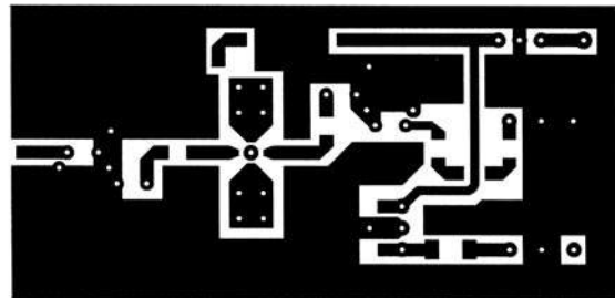
Dessin du circuit imprimé (double face).
