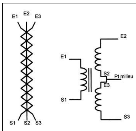
Transformateur large bande.
