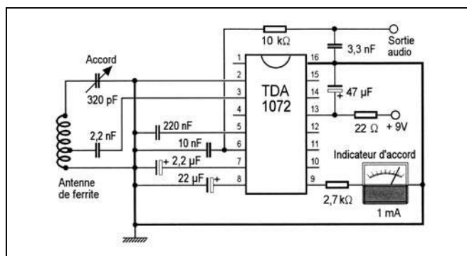
Fig. 1.— La section de fréquence intermédiaire du TDA 1072 étant utilisable jusqu'à 2 MHz, on peut l'employer pour un récepteur à amplification directe qui, malgré sa simplicité, est doté d'un commande automatique de gain.
