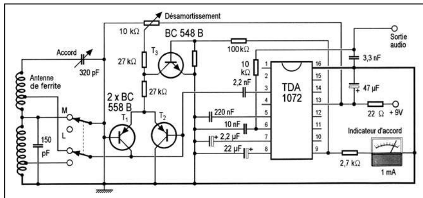
Fig. 3. – Lors de la réception d'un signal fort, on peut se permettre une bande passante plus large, et cela détermine une meilleure qualité d'audition. Une commande automatique maintient cette largeur de bande à sa valeur optimale et améliore ainsi agréablement le confort d'écoute.
