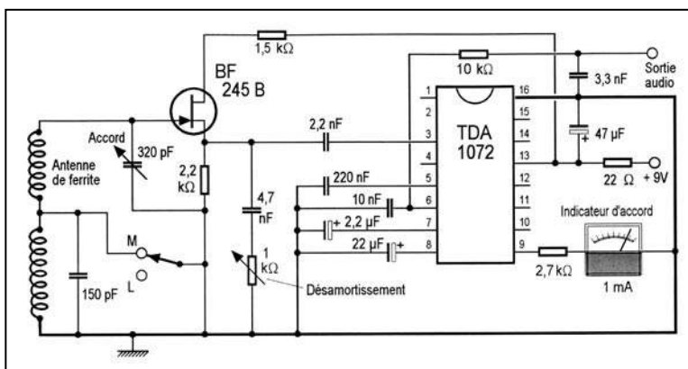
Fig. 2.— La compensation ajustable des pertes du circuit résonnant augmente la sensibilité tout en améliorant la sélectivité en imposant un filtrage plus étroit. La commutation des gammes se fait par le court-circuit de l'un des enroulements.
