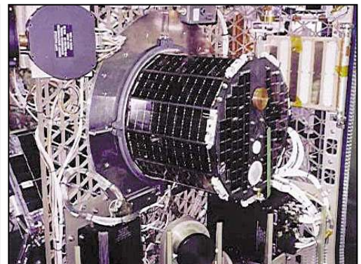
ASUSAT fixé sur JAWSAT.
