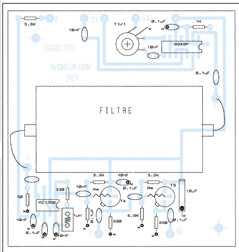
Implantation.4 Woblateur 0,5-45 MHz.
