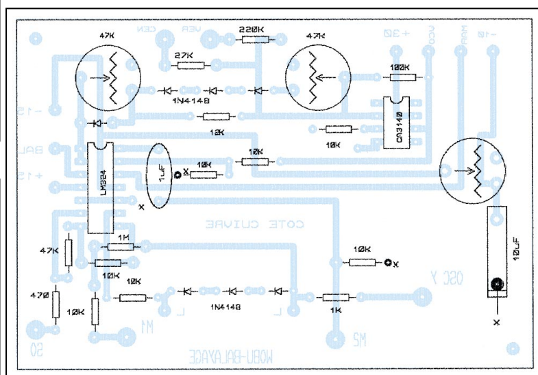
Implantation.5 Woblateur 0,5-45 MHz.
