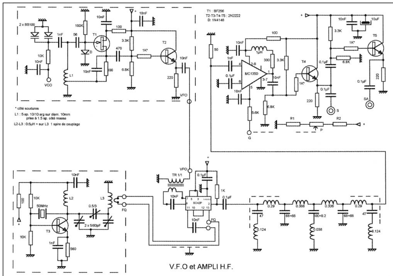
Synoptique.1 Woblateur 0,5-45 MHz.
