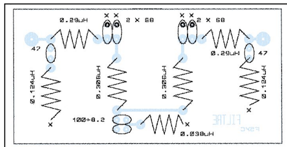
Implantation.3 Woblateur 0,5-45 MHz.
