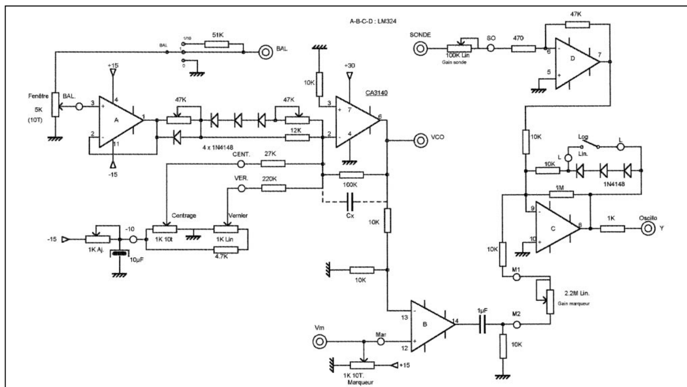
Synoptique.2 Woblateur 0,5-45 MHz.
