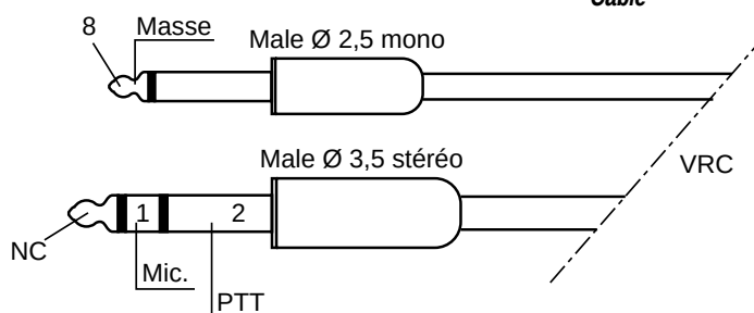
Câble
