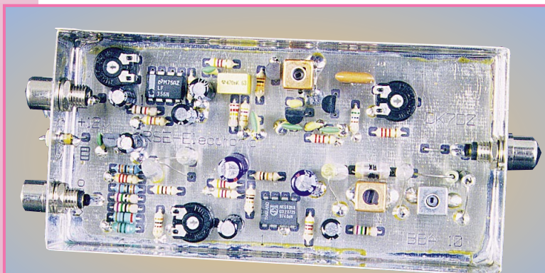
Modulateur audio + vidéo (RSE).
