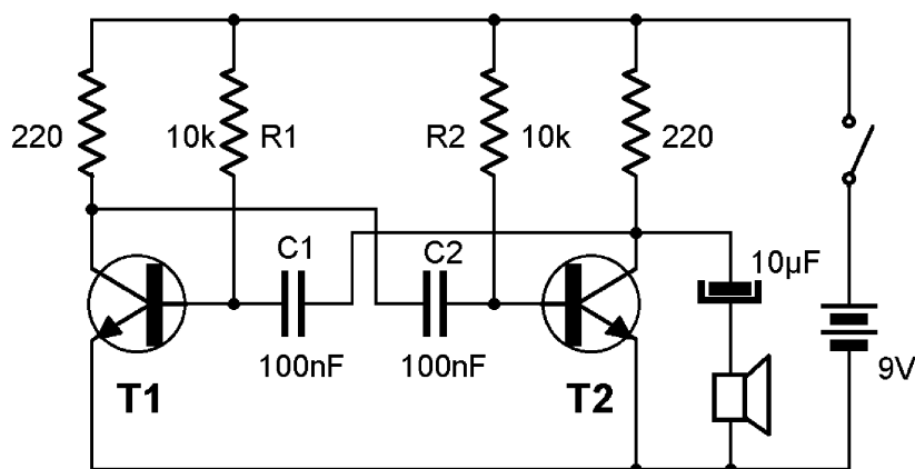
Figure 1 - Schéma d'un multivibrateur.
