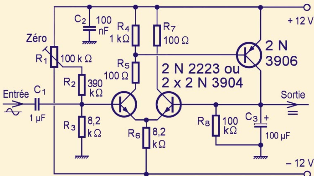
Figure 2 : La version discrète du redresseur de crête se distingue par une plus grande bande passante, mais présente une linéarité un peu moins bonne.
