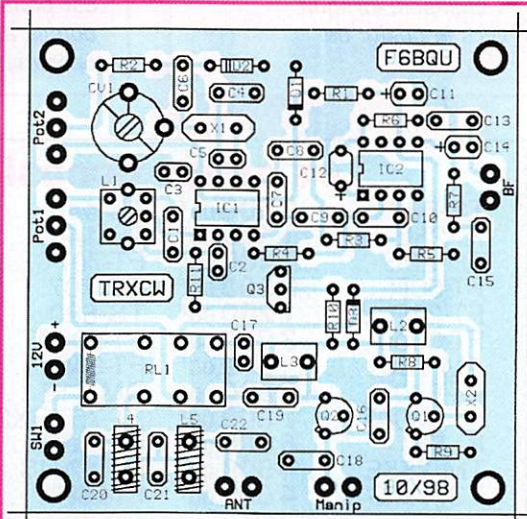
Implantation du TRX 80 m CW.
