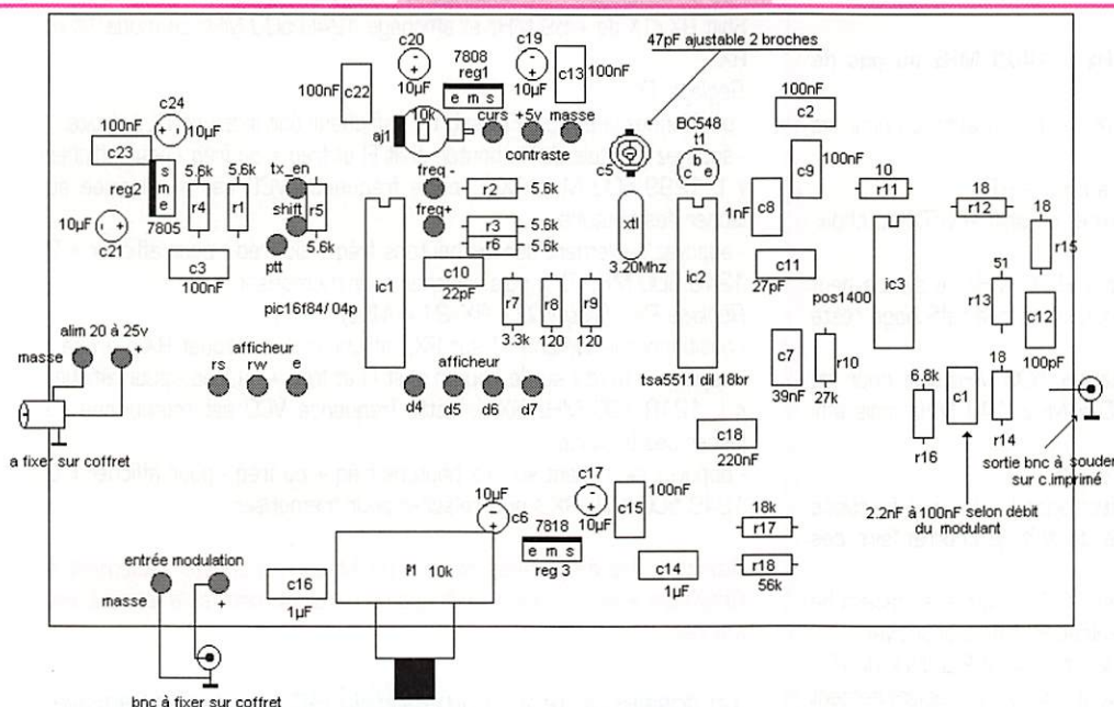
Géné 1.2 GHz. Implantation. Vu côté composants.
