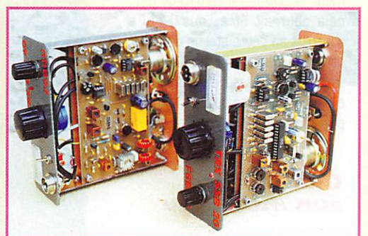
A peine plus compliqué : E/R BLU réalisé par F6BQU.
