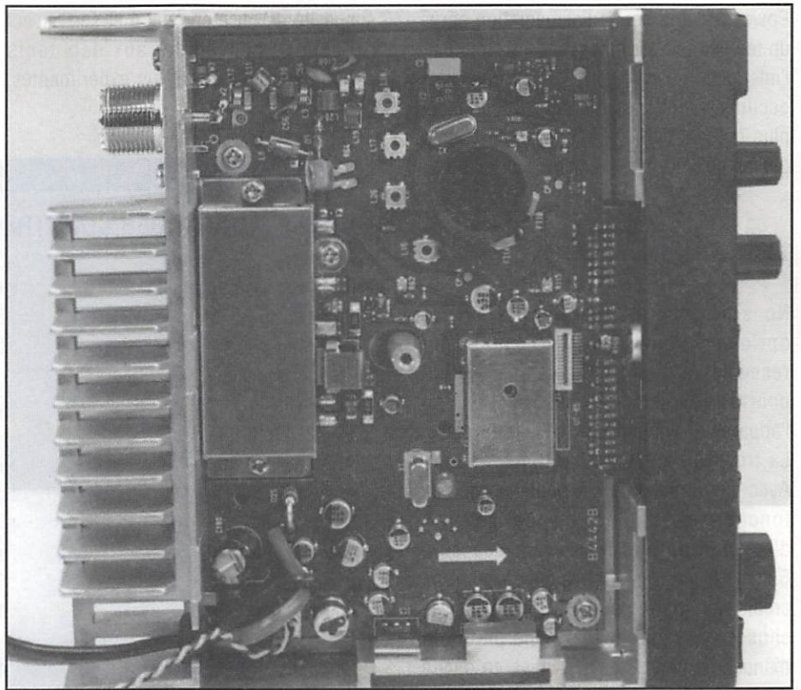
Une platine aux composants fort dispersés !
