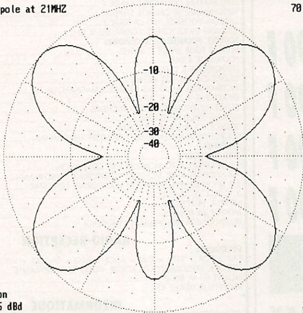
Figure 2 - Diagramme de rayonnement vertical sur 21 MHz d'un dipôle 40 m.
