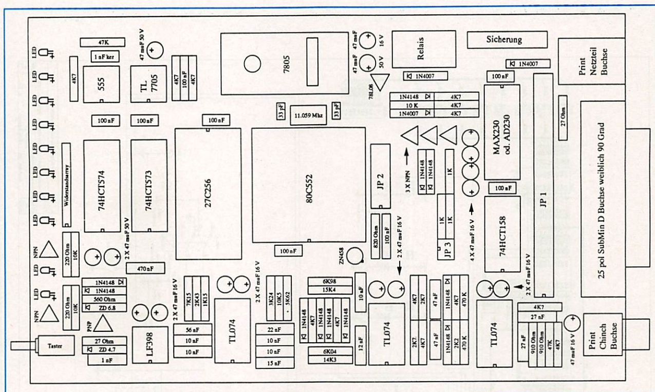
Figure 4 – Schéma d'implantation.
