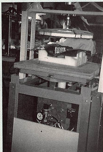
Banc testant la résistance aux vibrations.
