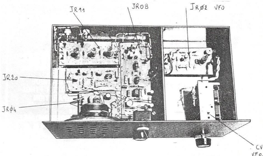
Récepteur monobande 7 MHz constitué des modules JR 11 + JR 08 + JR 04. Montage effectué dans une école de Neukirchen (RFA)
