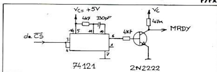
Figure 5 — Ralentisseur d'horloge
