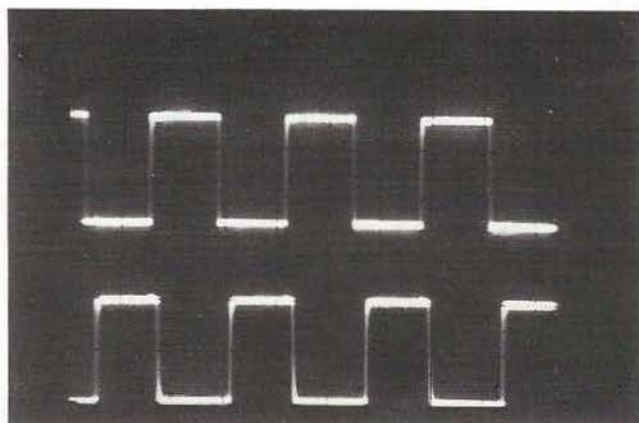
PHOTO 4: F_i \cong F_o + F_c . Le déphasage entre V_i et V_r atteint presque \pi . La valeur moyenne de V_1 , sortie du OU exclusif atteint V_{DD} .
