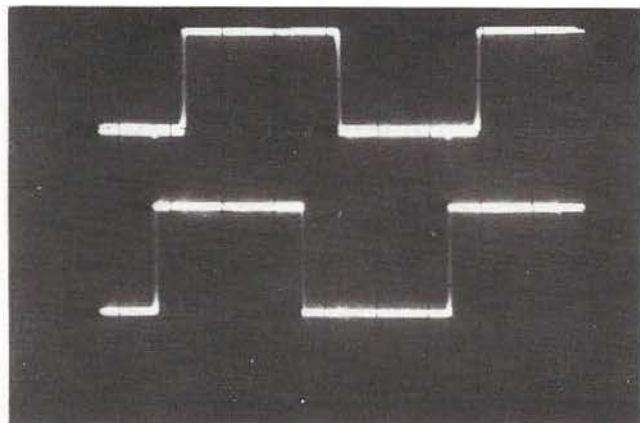
PHOTO 3: mêmes légendes que la photo 2. Ici F_i \cong F_o - F_c . Il y a un déphasage presque nul entre V_i et V_r . La valeur moyenne de V_1 est presque nulle.
