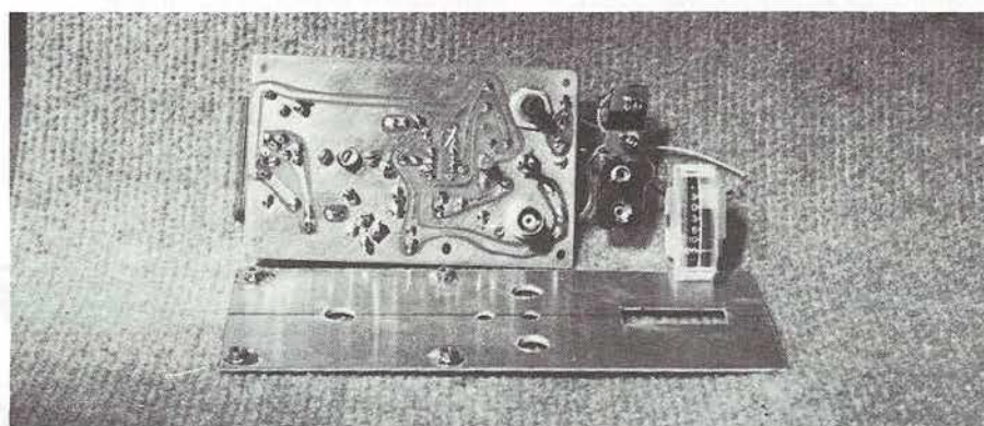
Photo 2: C1 côté cuivre et préparation de la face avant.
