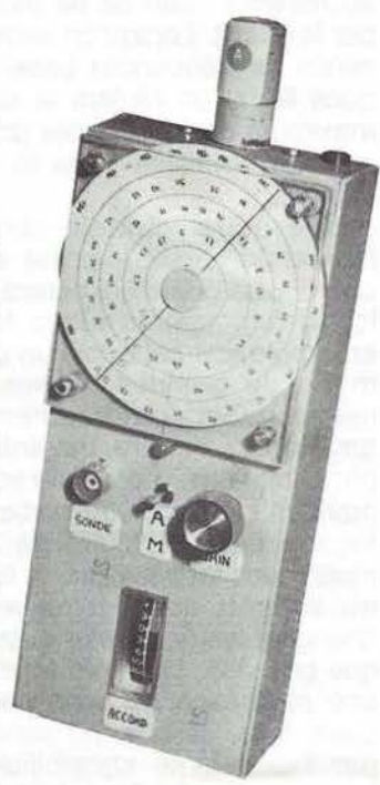
Photo 6: L'appareil terminé.
