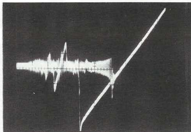
PHOTO 6: Agrandissement de la précédente, le balayage n'atteignant plus F_0 + F_1 .
