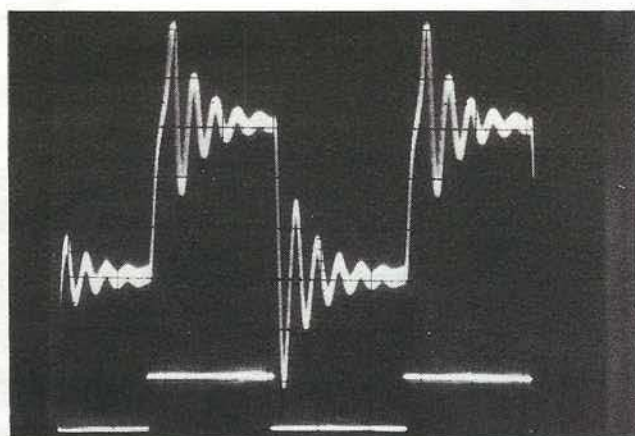
PHOTO 7: F_1 proche de F_0 + F_c .
