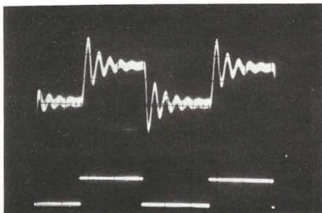
PHOTO 1 (0,5 ms/carreau): Réponse linéaire de la boucle (en haut) à un échelon de fréquence (en bas) D = \frac{a}{b} = 0,7 ; \tau \approx 600 \mu s
