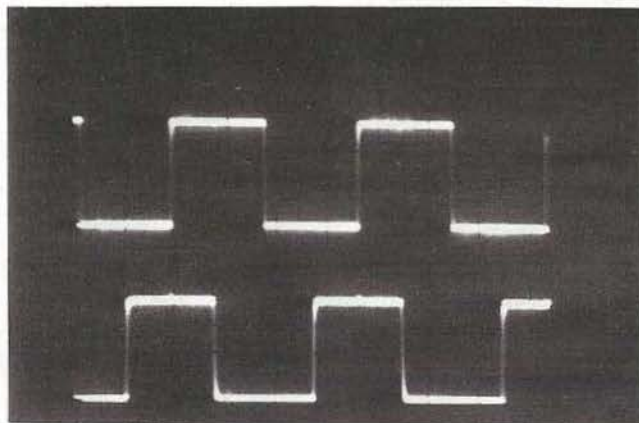
PHOTO 2: F_i \cong F_o . La valeur moyenne de V_1 vaut 0,5 V_{DD} V_i en bas 5V/cm 5 \mu s/carreau V_r en haut Il y a un déphasage de \pi/2 entre V_i et V_r .
