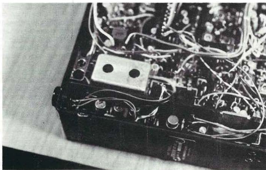
INSTALLATION DU CIRCUIT IMPRIME A L'EMPLACEMENT DE L'ANTENNE TELESKOPIQUE.
