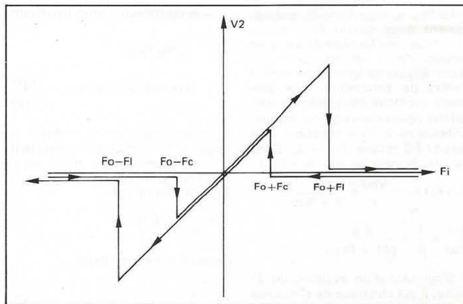
FIGURE 6: CARACTERISTIQUE DE TRANSFERT D'UNE PLL.
