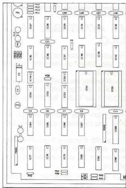
- plan d'équipement
