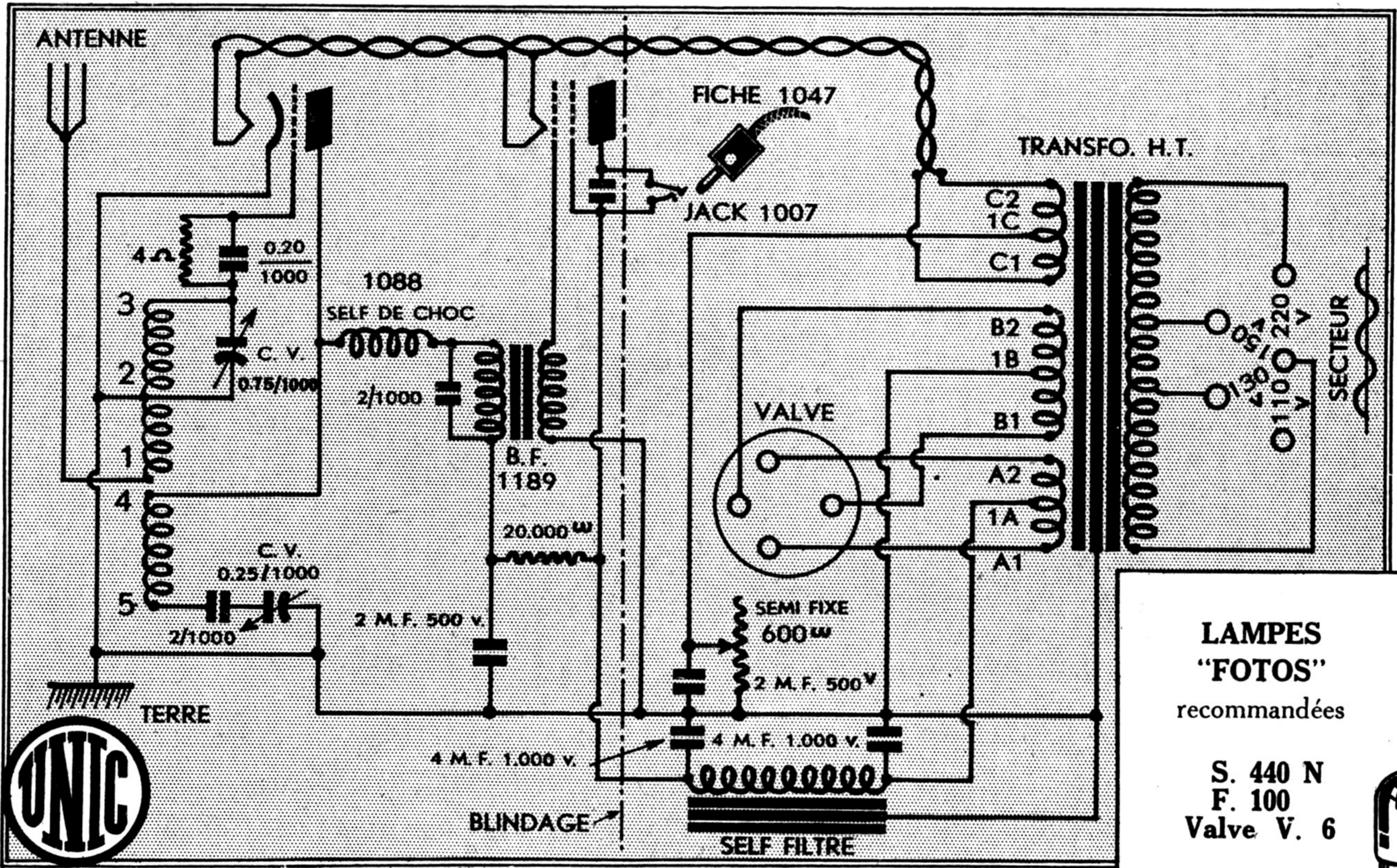
POSTE 2 LAMPES "SECTEUR" 1 DÉTECTRICE. 1 BASSE FRÉQUENCE
