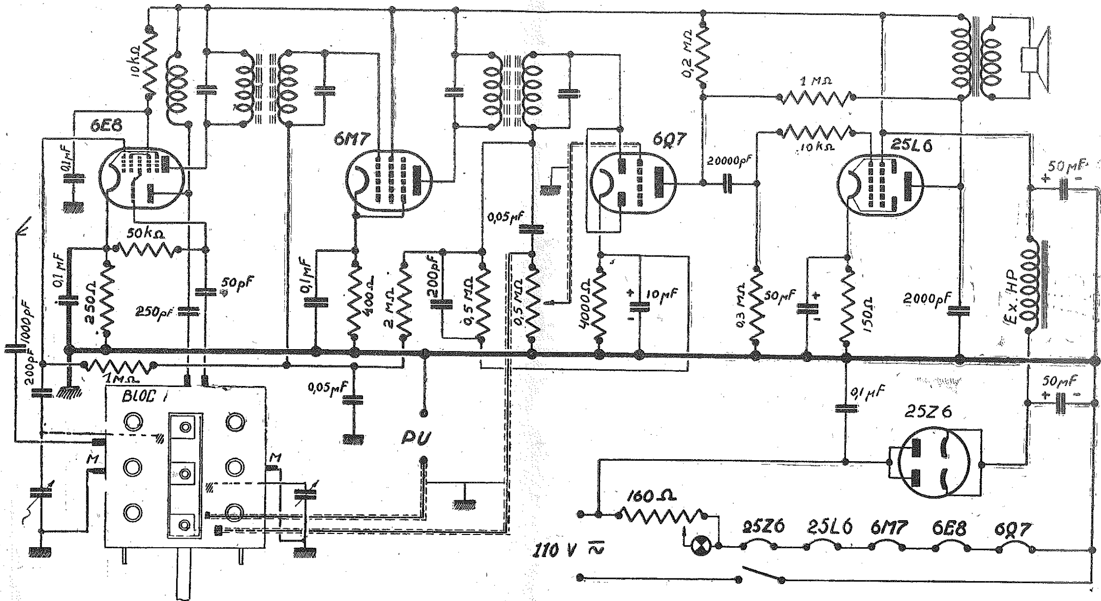
Schéma technique SLAM-TC5 Américain
