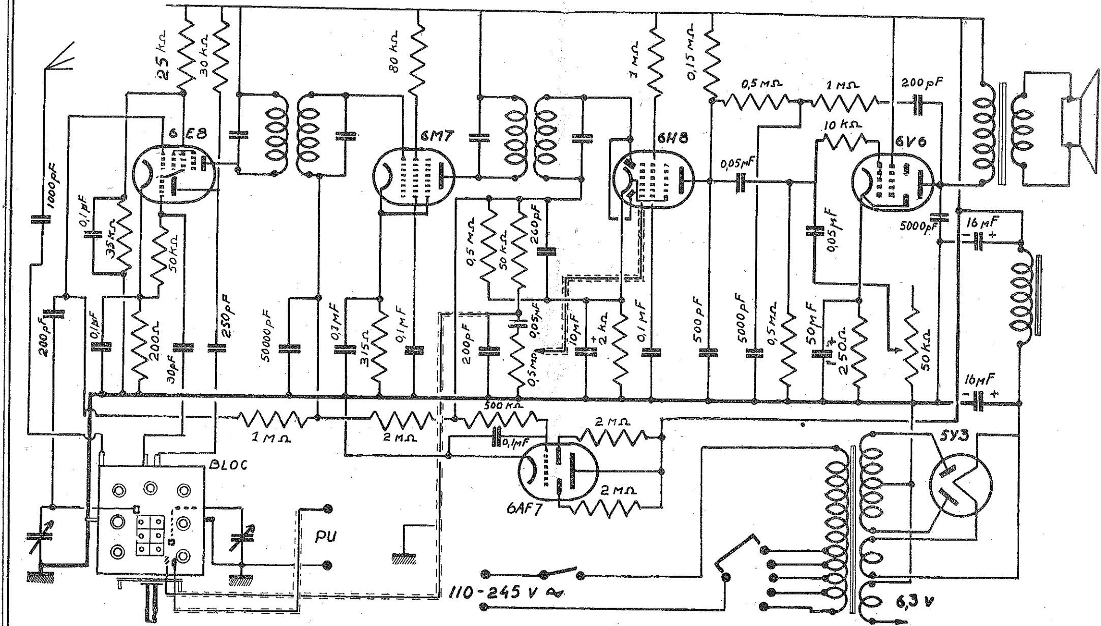
Schéma technique SLAM-A6 Américain
