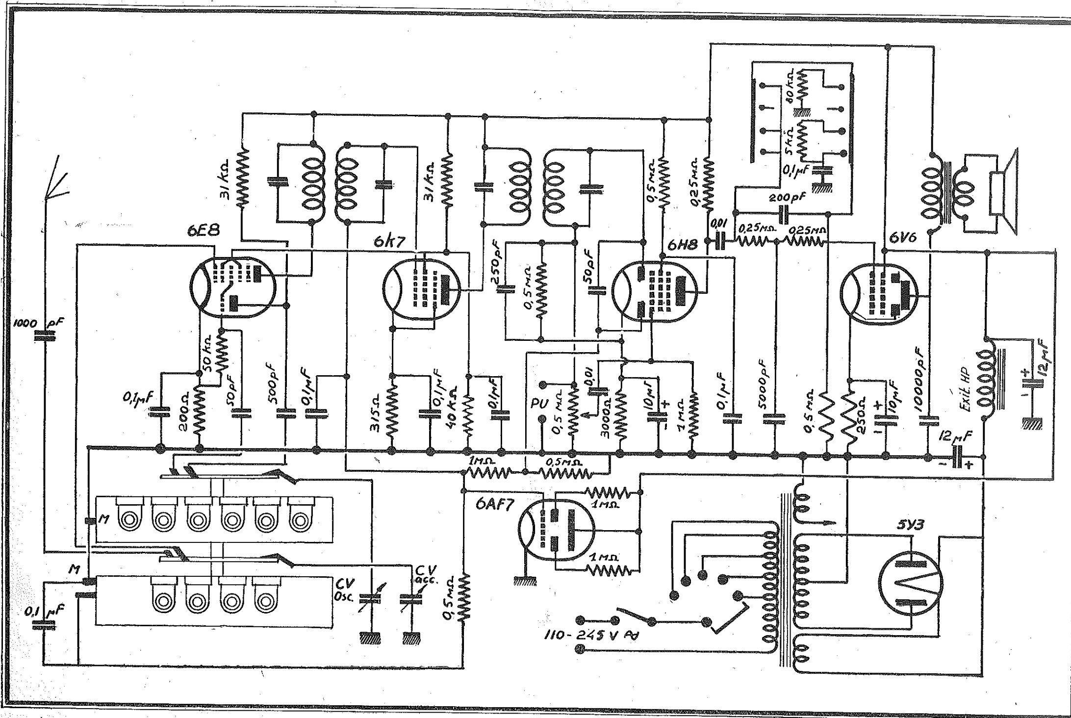
Schéma technique SLAM-6 4 gammes
