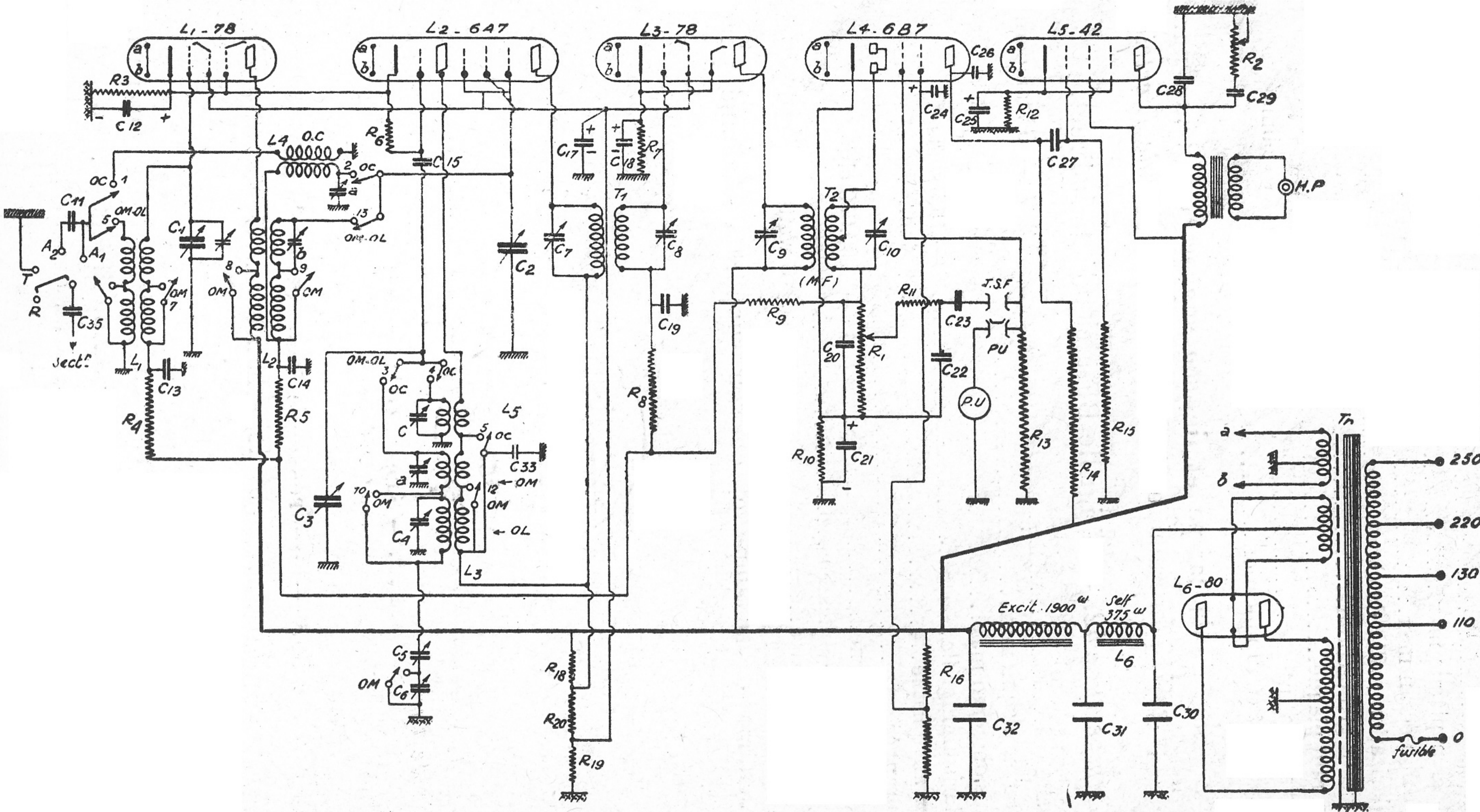
Fig. 3. — Schéma du Super-Synchrovox 6-35.
